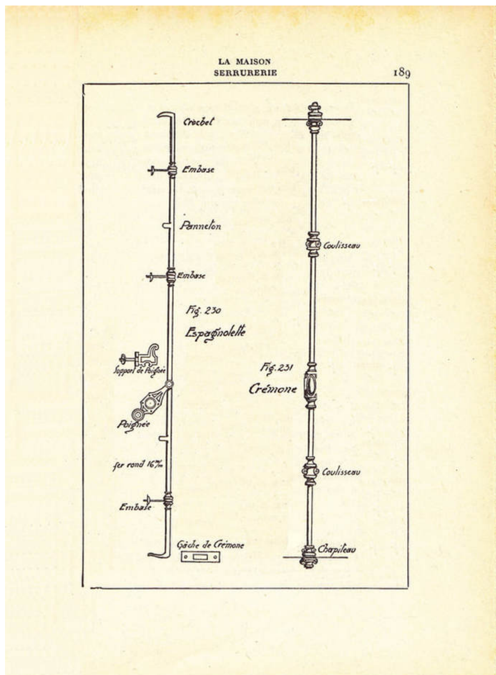
afb. 9.4.6 - 14 Het verschil tussen espagnolette en crémone. In het Nederlands wordt een crémone soms ook krukespagnolet genoemd. Een pompespagnolet is een crémone die niet door een draaigreep maar door een op en neer zwenkende 'pompende' hendel bediend wordt.
