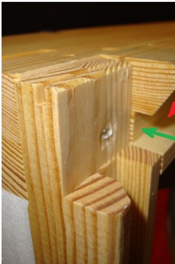
afb.06.5.5 - 3 De twee mogelijkheden afwerkingsplaten te plaatsen
