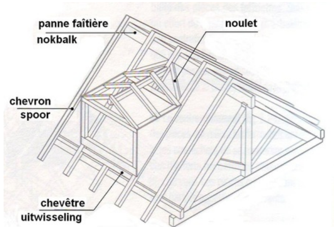
afb. 06.4 - 35 (schets uit het boek van Gérard Calvat: La maison de A à Z)
